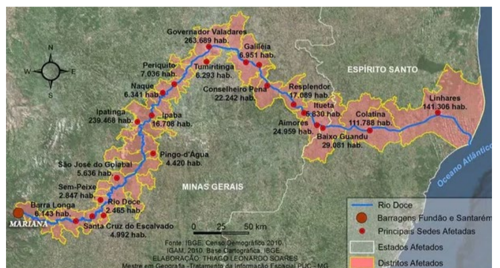
O caminho da Lama: de Mariana (MG) a Linhares no Espírito Santo
